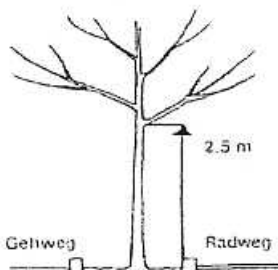
Lichttraum-Profil... ... an Geh- und Radwegen
