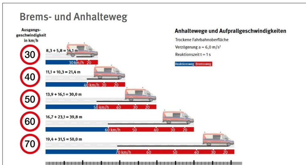
Abbildung 18: Brems- und Anhalteweg bei unterschiedlichen Geschwindigkeiten
