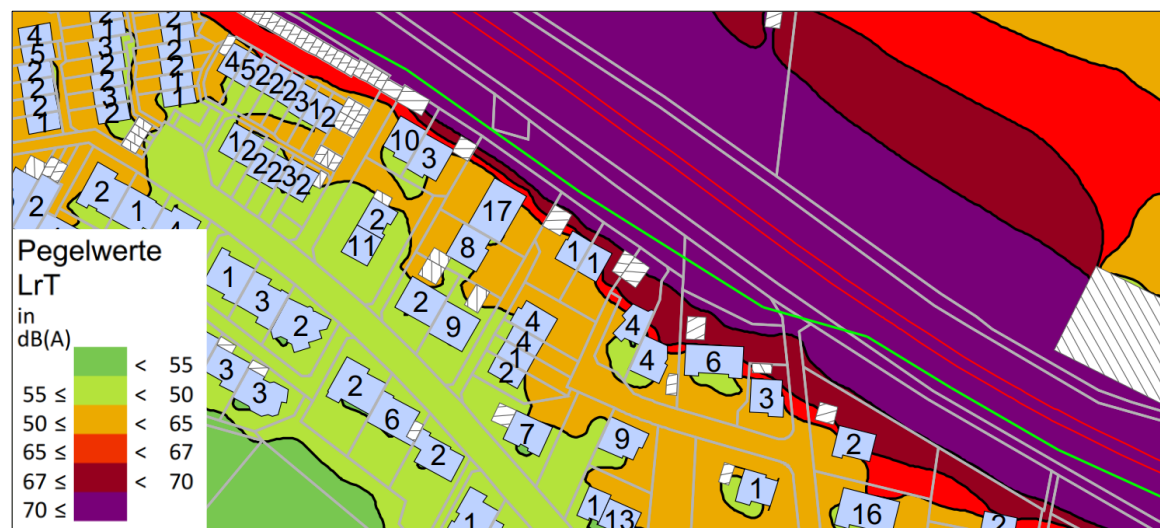
Abbildung 4: Auszug Rasterlärmkarte Tag
