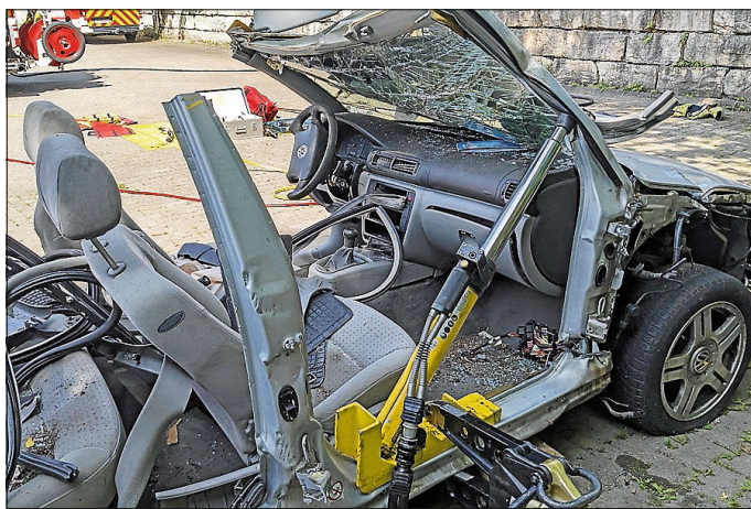
Mit einem hydraulischen Stempel und einem Schwelleraufsatz wird der Zugang vergrößert Fotos: FF Schwieberdingen
